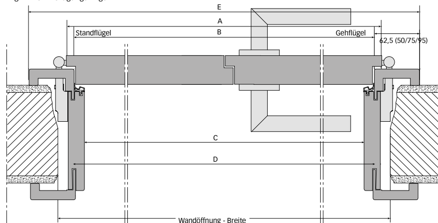
2-flg. Einzelerstellungszarge
